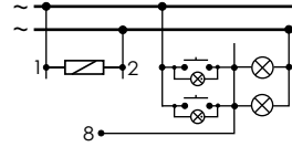
instalacja 3-przewodowa
