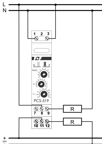
Przykładowy układ zasilania napięciem 230V przekaźnika sterującego odbiornikiem zasilanym napięciem 230V i 24V.
