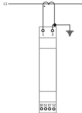
Pośredni pomiar natężenia prądu z wykorzystaniem przekładników prądowych.
