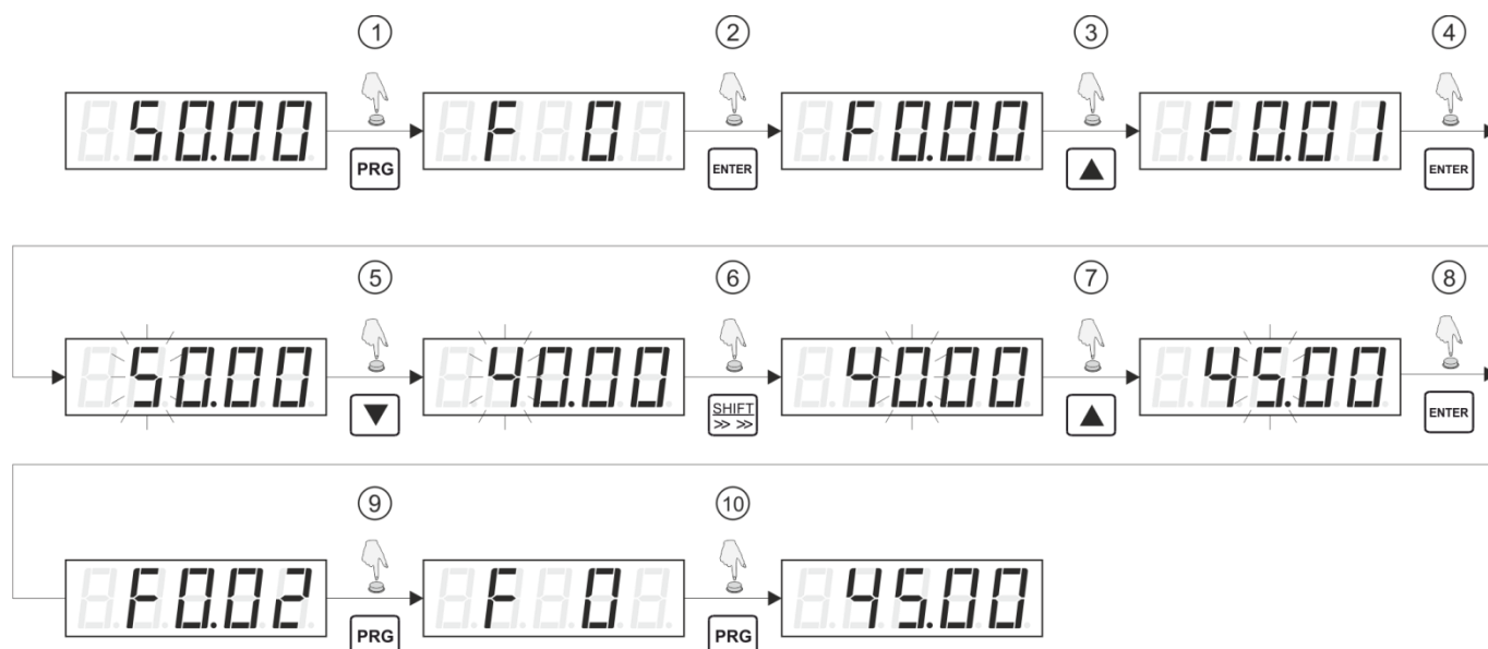
Rys. 10 Przykład postępowania – zmiana częstotliwości zadanej
