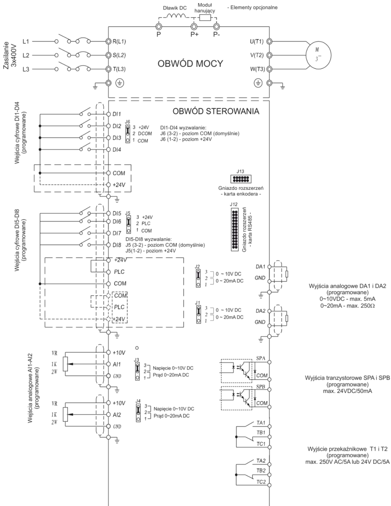
Rys. 5) Schemat podłączenia falownika FA-3X220
