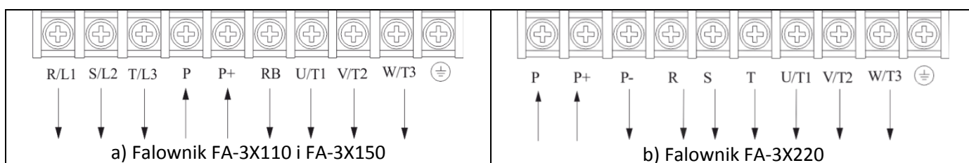
Rys. 6) Listwa zaciskowa do podłączenia obwodów mocy
