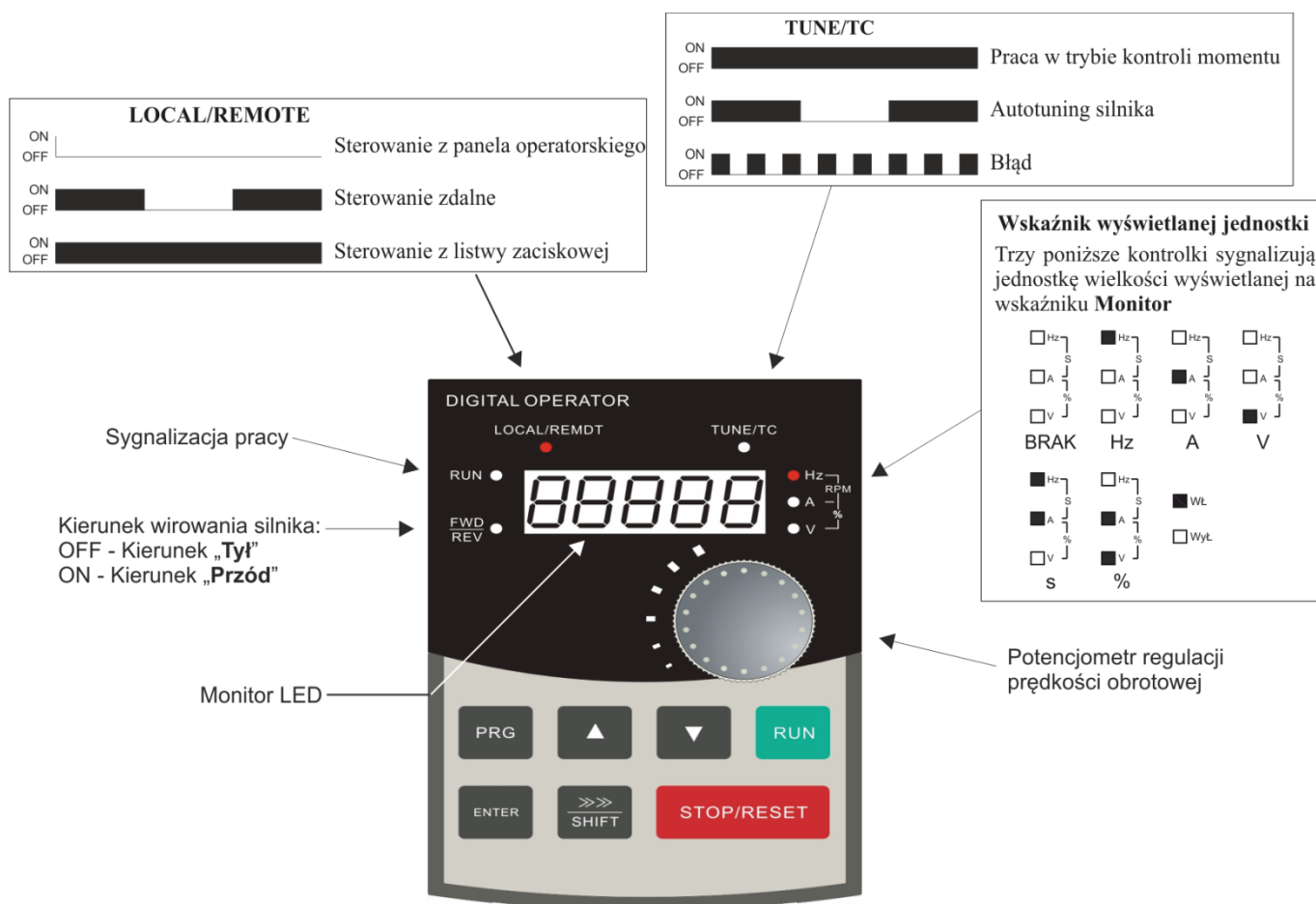
Rys. 8) Panel sterowniczy – elementy sygnalizacyjne
