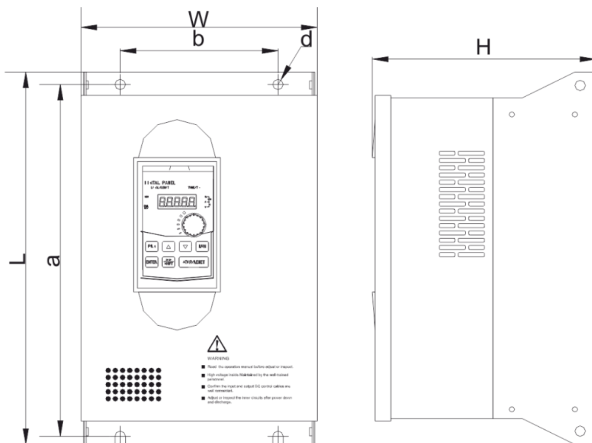
Rys. 11) Wymiary falownika i rozmieszczenie otworów pomiarowych
