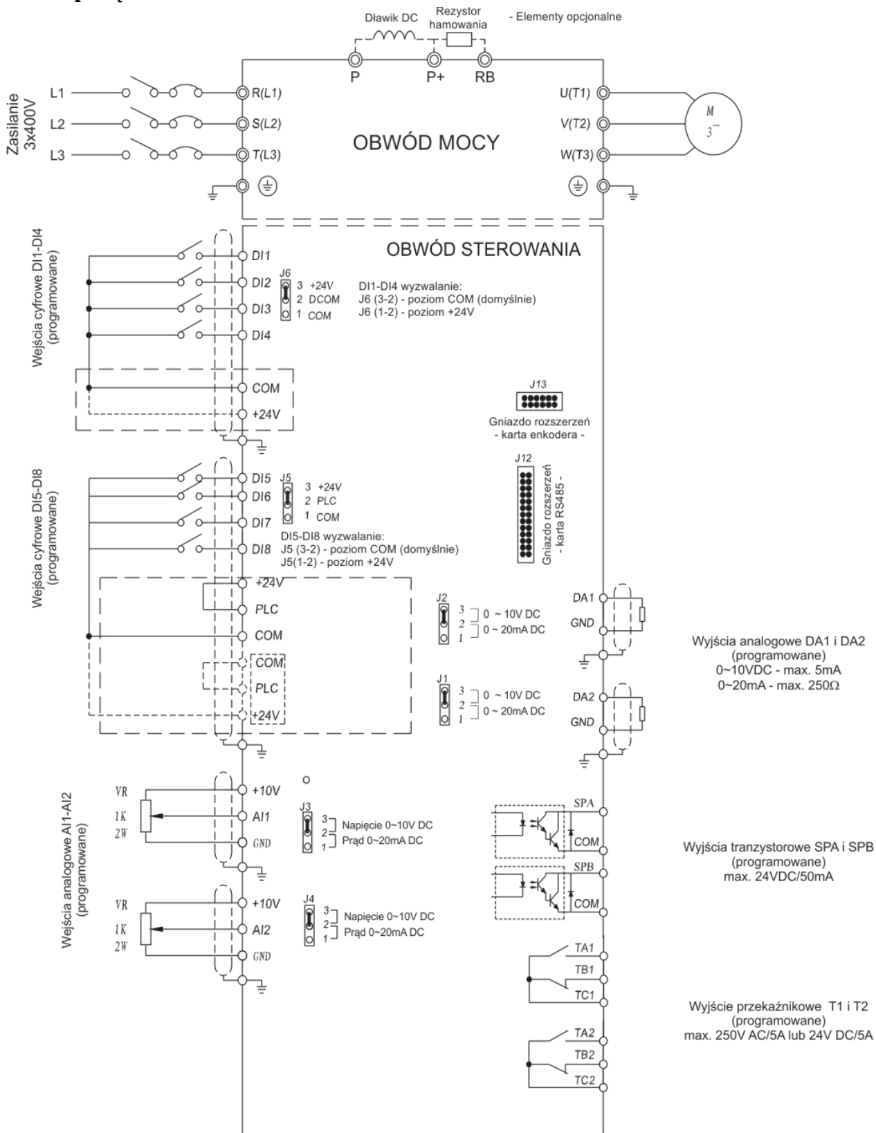
Rys. 4) Schemat podłączenia falownika FA-3X110 i FA-3X150
