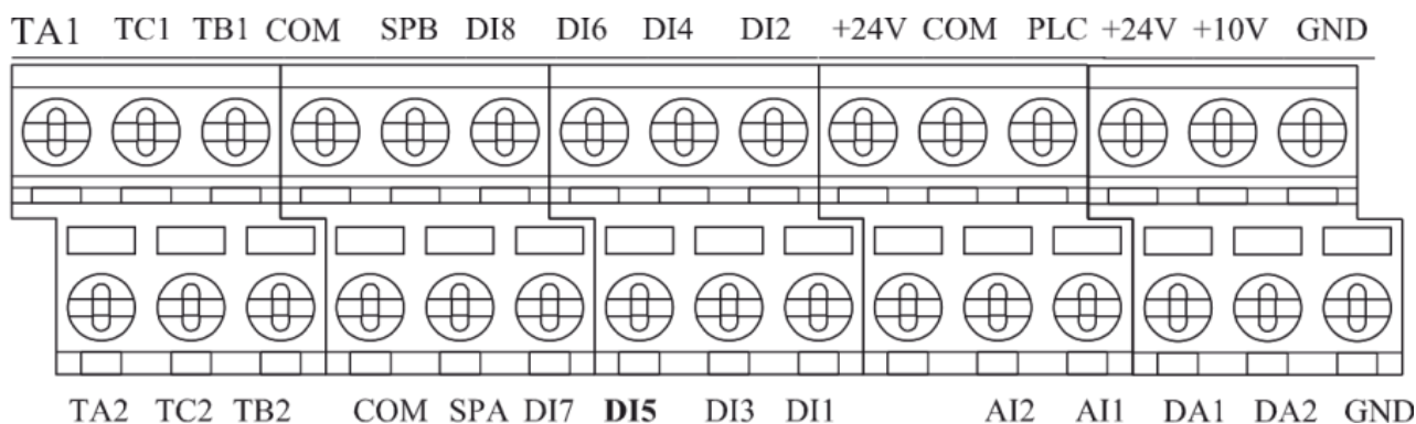
Rys. 7) Listwa zaciskowa obwodów sterowniczych
