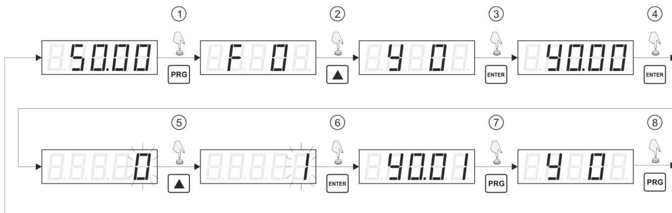
Rys. 9) Przykład postępowania – przywrócenie konfiguracji domyślnej
